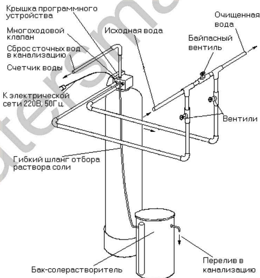
Схема монтажа установки
